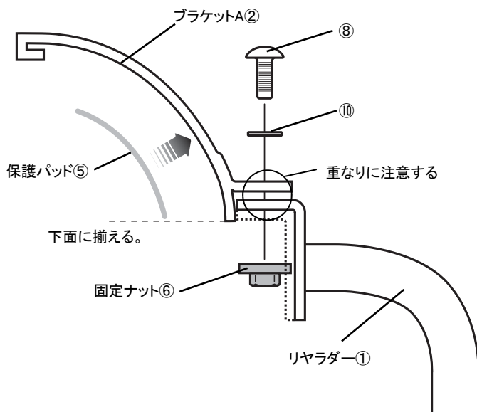
穴位置を合せ、ブラケットA②が垂直になる様配置し、ボディ側に保護シート④を、ブラケットA②の方へ保護パッド⑤を貼り付ける。
