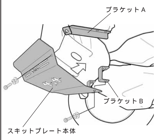
図3 スキットプレート本体の取付
