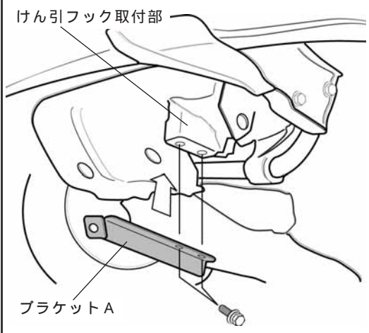
図1 ブラケットAの取付 (助手席側)
