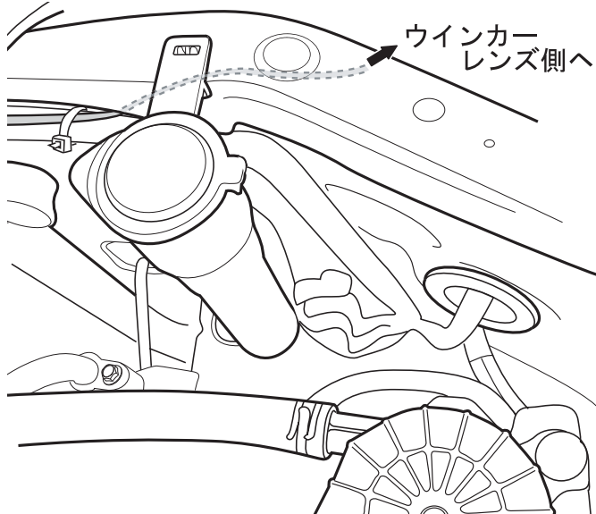
右ヘッドライト裏側部
