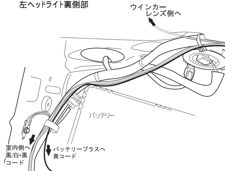
室内側へ配線
