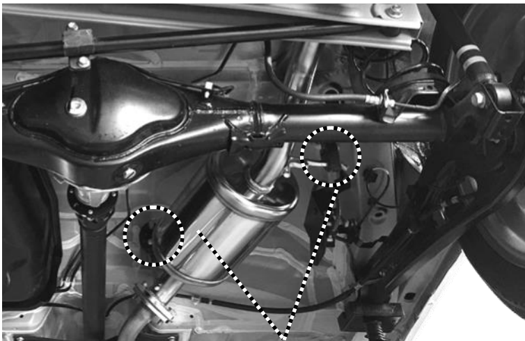
純正パイプサポート 再使用
